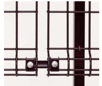
調整継手(下)
